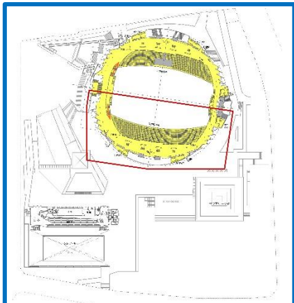
メインアリーナ棟 2階平面：南側
