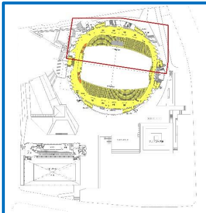
メインアリーナ棟 2階平面：北側
