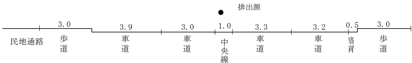
図2. 1-2 予測地点の道路断面(No. 1)
