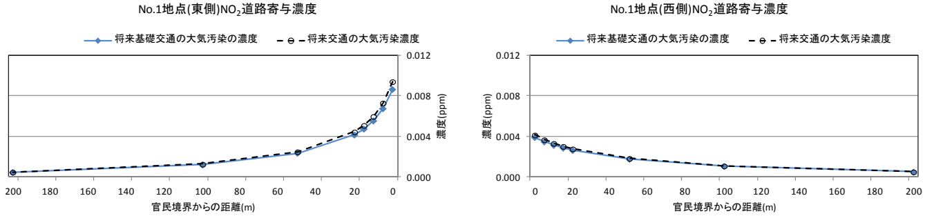
図2.1-6(1) 工事の施行中における二酸化窒素寄与濃度の距離減衰 (No. 1)
