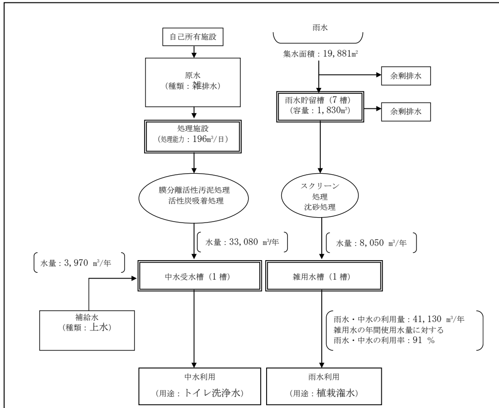
図 9.9-1 雨水・循環水（中水）利用の流れ
