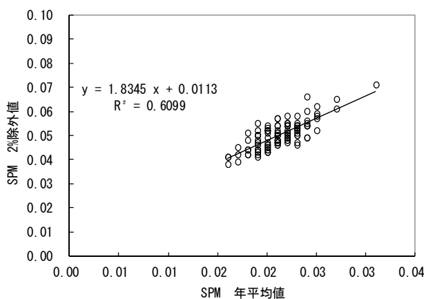
図2.1-7(2) 浮遊粒子状物質の日平均値の年間2%除外値への変換式相関図(一般大気環境測定局)
