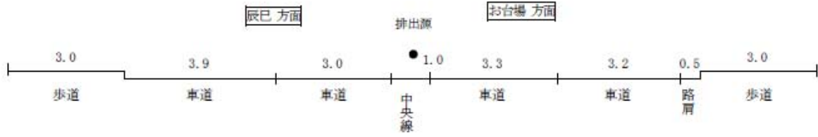
図2.1-3(1) 予測地点の道路断面 (No. 1)
