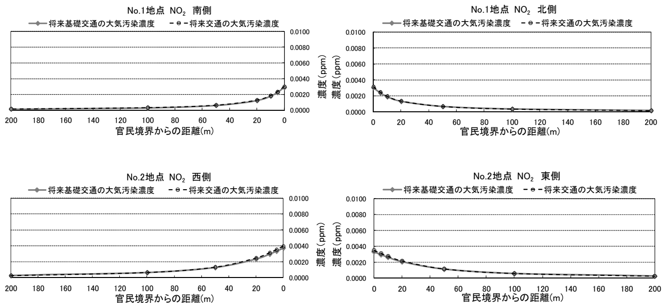
図2.1-6(1) 工事の施行中における二酸化窒素寄与濃度の距離減衰 (No. 1~2)
