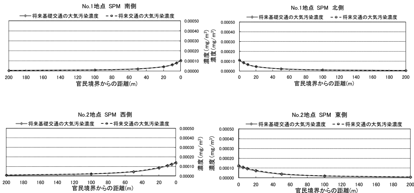
図2.1-6(2) 工事の施行中における浮遊粒子状物質寄与濃度の距離減衰 (No. 1~2)
