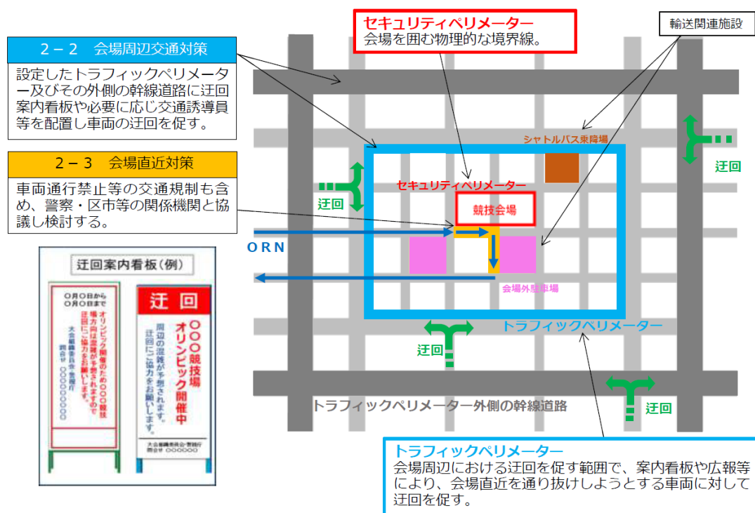
図 4.2-5 競技会場周辺の交通対策のイメージ図
