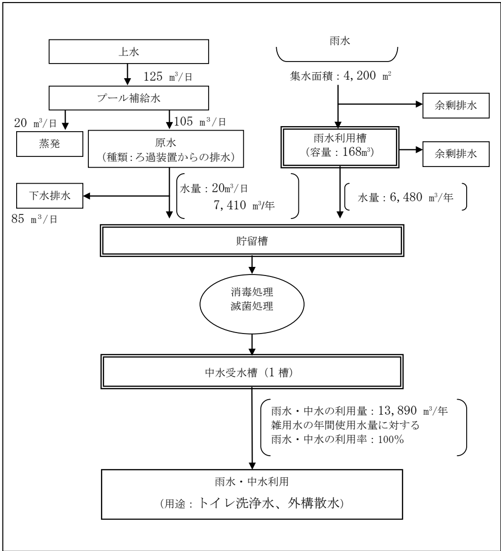
図 9.10-1 雨水・循環水（中水）利用の流れ
