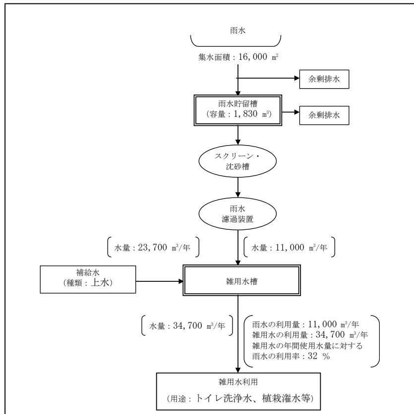
図 9.9-1 雨水利用の流れ
