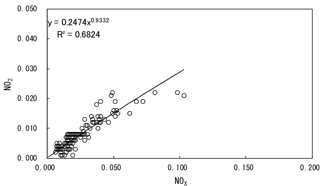
図2.1-5 二酸化窒素 ( \text{NO}_2 ) の変換式の相関図
