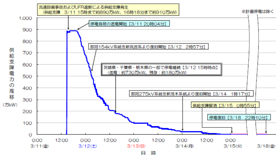
図9.15-1 東日本大震災による東京電力（株）エリアにおける停電の推移
