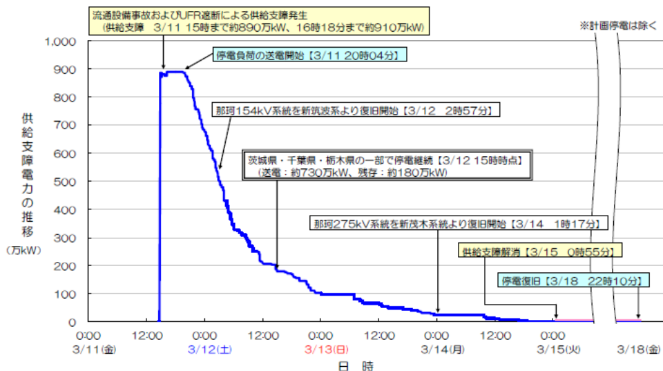
図9.10-1 東日本大震災による東京電力(株)エリアにおける停電の推移
